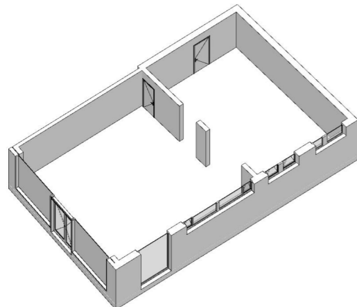
AXONOMETRIE PROVOZOVNY
